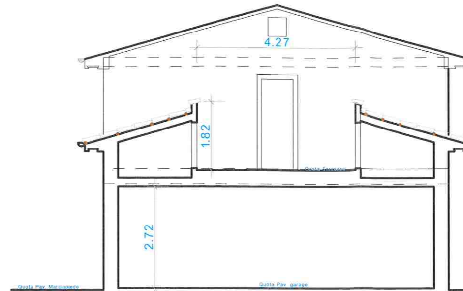
Sezione A-A ATTUALE PROPRIETA' BRESSAN
