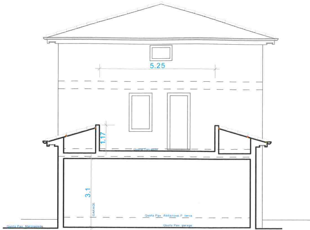
Sezione A-A ATTUALE PROPRIETA' DUGATTO
