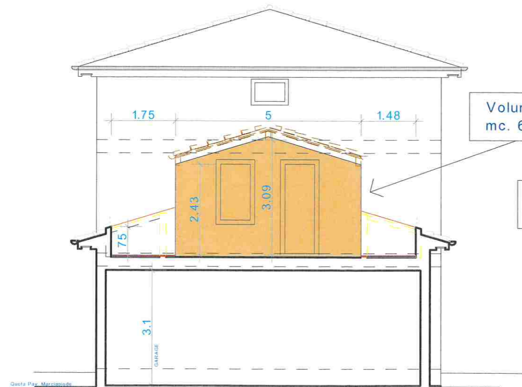
Sezione A-A FUTURO
