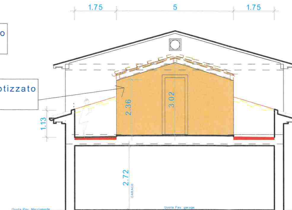
Sezione A-A FUTURO
